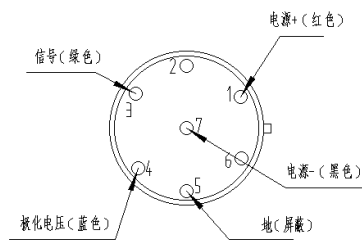
LEMO头，从插针面看入
